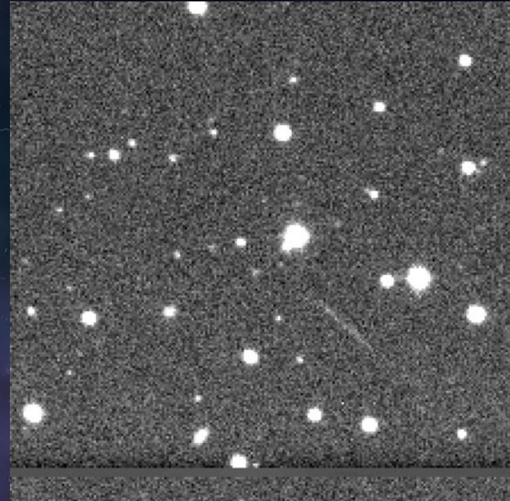
Objav near-Earth asteroid 2023 BE2 Foto: K. Sárnecky & Objav : Š. Kürti
